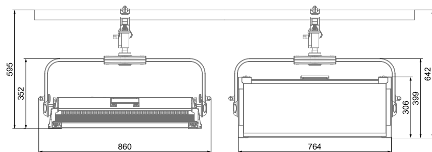
吊挂尺寸图
