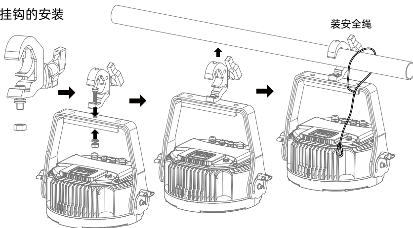
吊挂尺寸图
